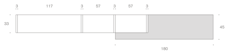
SP019 L/W 363 | H 183 | P/D 33-45
