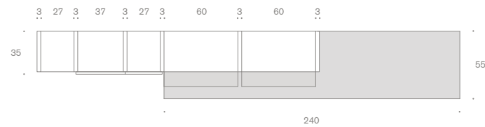
SP023 L/W 343 | H 163 | P/D 35-55
