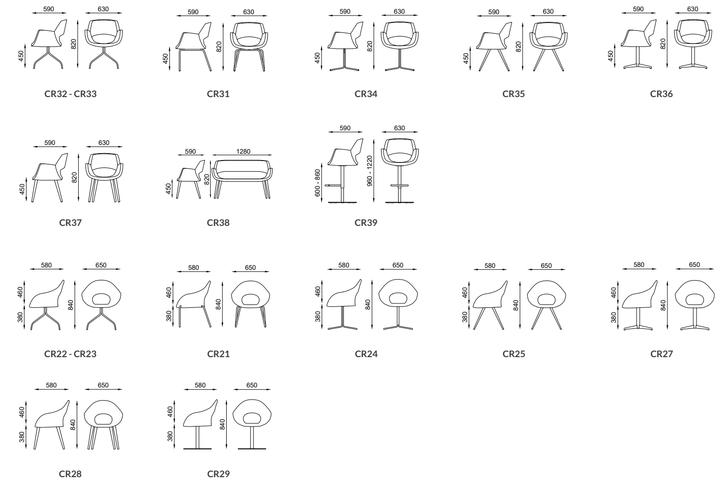
DETTAGLI / DETAILS
